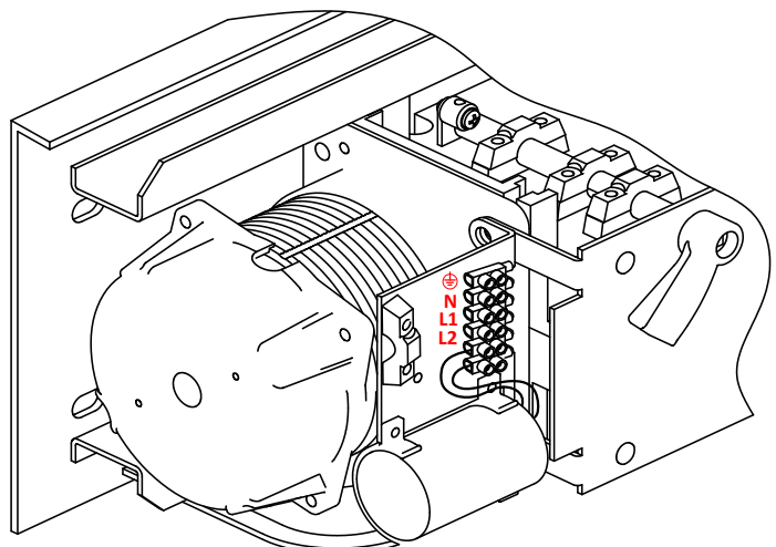
Рисунок 16. Подключение привода ASW4000 к модулю. Перемычки XN1 и XN2 модуля должны быть сняты (контакты разомкнуты)!
