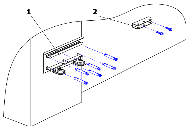
Рисунок 10. Установка креплений
